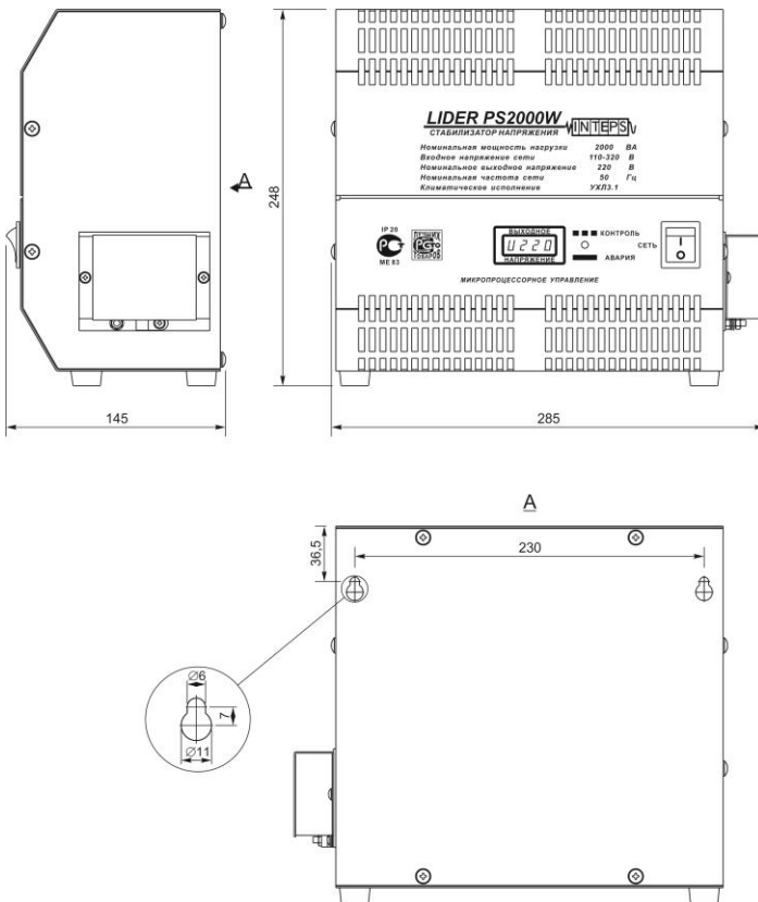
Габаритные и установочные размеры стабилизаторов напряжения переменного тока LIDER PS1200W-50
