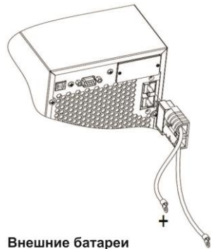
Рисунок 5а. Подключение батарейного кабеля к ИБП исполнение ДТ.
