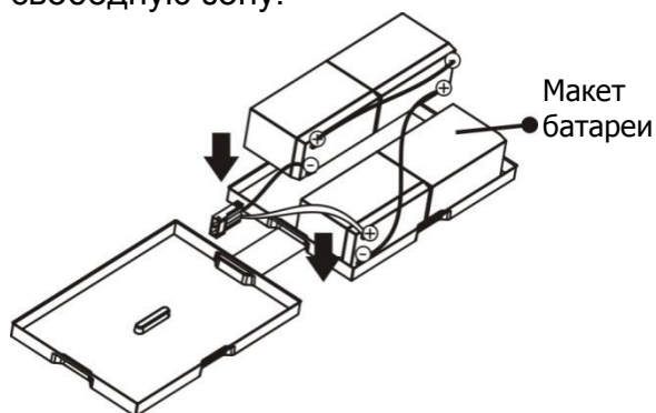
Рисунок 9. Порядок сборки комплекта из трех батарей.
