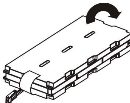
Рисунок 11. Порядок сборки комплекта из шести батарей.
