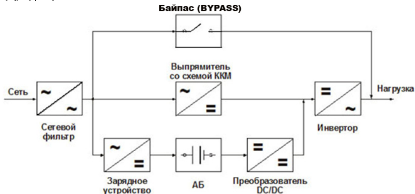
Рисунок 1. Структурная схема ИБП.
