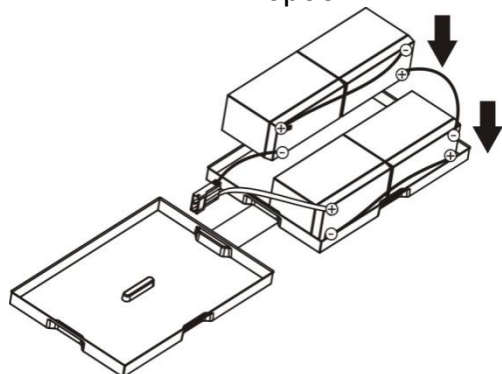
Рисунок 10. Порядок сборки комплекта из четырех батарей.
