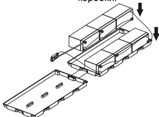
Рисунок 11. Порядок сборки комплекта из шести батарей.
