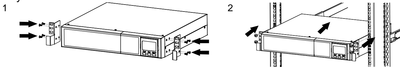
Рисунок 3. Установка в 19 дюймовую стойку.
