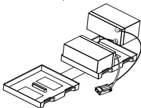
Рисунок 8. Порядок сборки комплекта из двух батарей.
