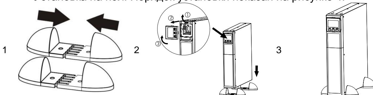
Рисунок 4. Установка в 19 дюймовую стойку.
