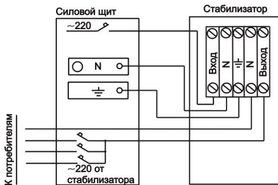
Рисунок 2 – Схема электрических соединений
