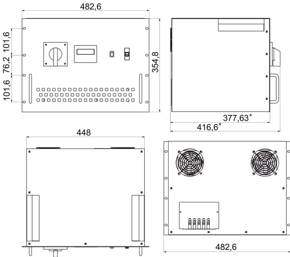
Габаритные и установочные размеры стабилизатора напряжения переменного тока LIDER PS1000SQ-R-15
