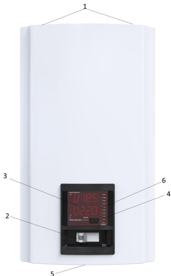
Рис.1 Внешний вид стабилизатора
